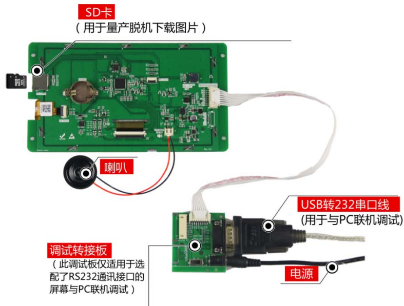
图 1-5 调试工具图
