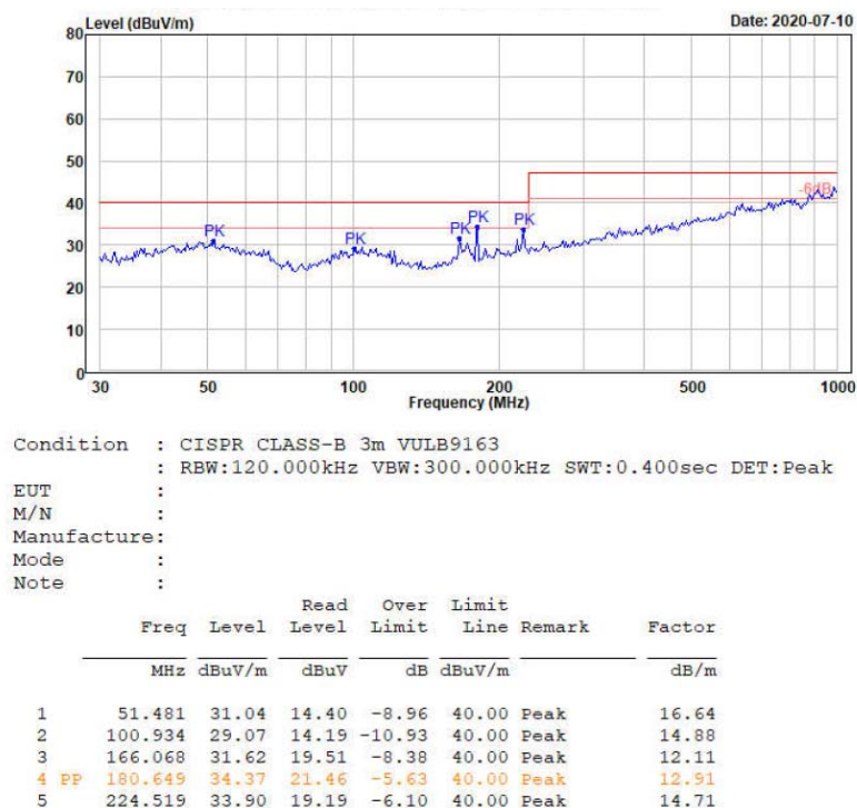
图 3-6 辐射测试水平方向
