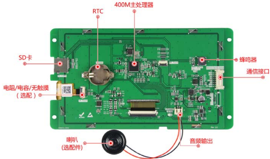
图 1-4 硬件配置图
