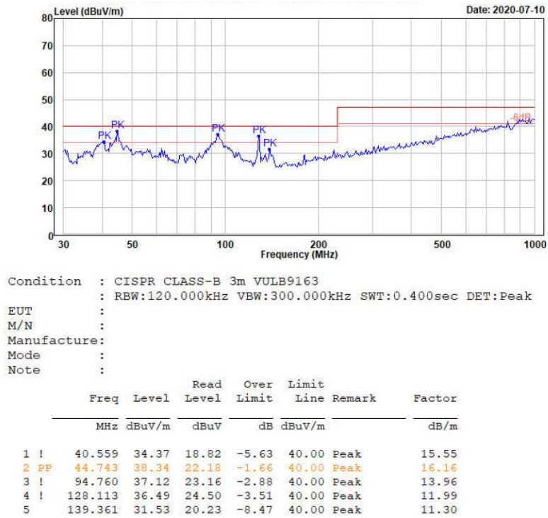
图 3-7 辐射测试垂直方向
